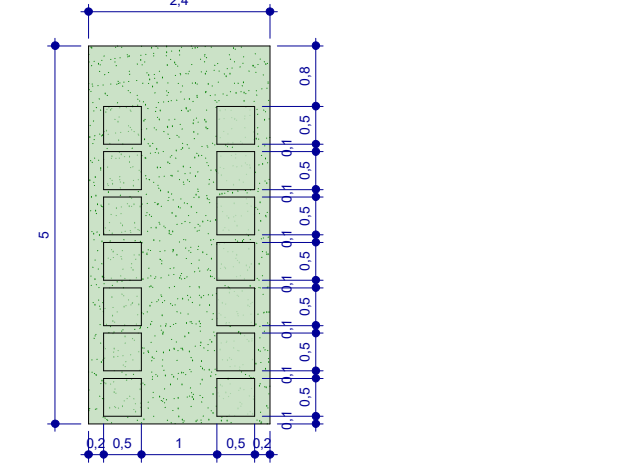
DETALHE - VAGA VISITANTE ESC.: 1:100
