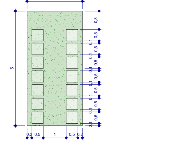
DETALHE - VAGA PERMEÁVEL ESC.: 1:100
