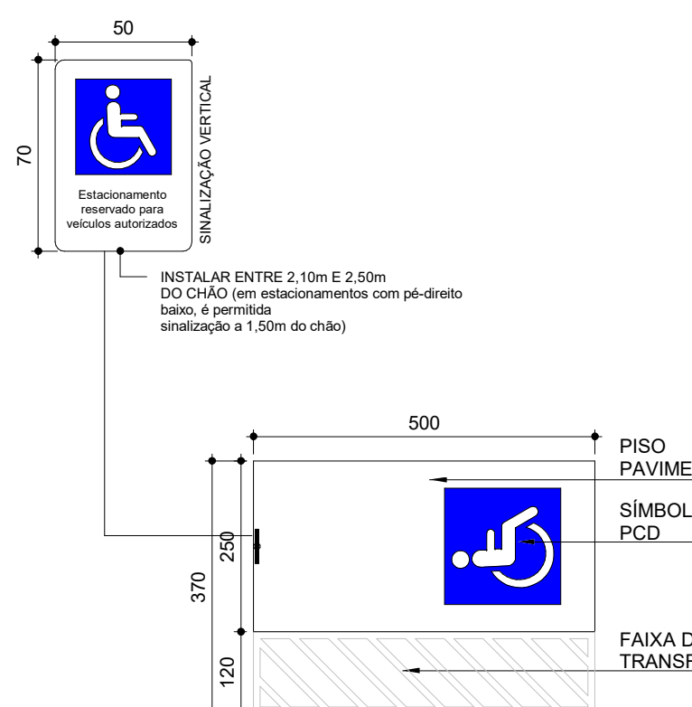
DETALHE - VAGA PCDD ESC.: 1:100
